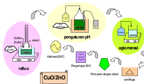
Gambar 2. Preparasi katalis
