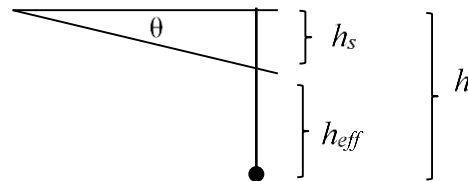
Gambar 5. Kemiringan permukaan dan kedalaman efektif.
