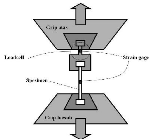
Gambar 2 – Konfigurasi Pengujian
