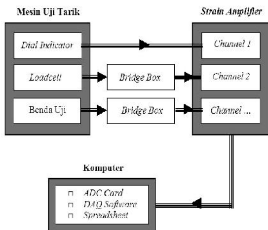
Gambar 3 – Instrumentasi Percobaan
