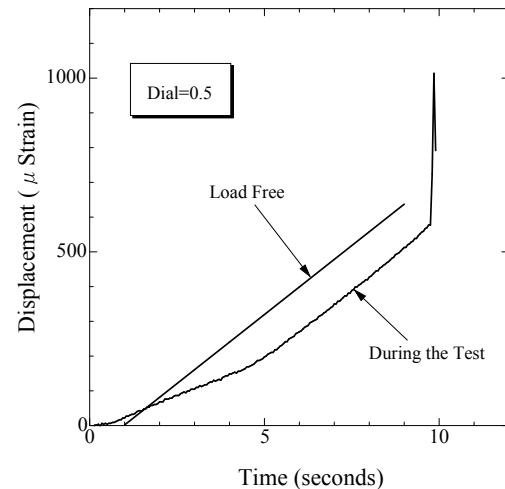
Gambar 6 – Hubungan antara Pergeseran Crosshead dan Waktu pada Kondisi Tanpa Beban dan Selama Pengujian dengan Posisi Dial 0.5
