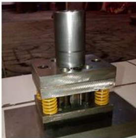
Gambar 6. Press tool
