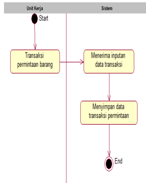
Gambar 4. Activity Diagram Menerima dan Menyimpan Transaksi Permintaan Barang.
