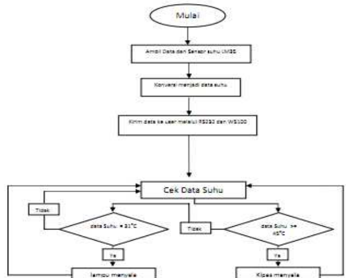
Gambar 9. Perancangan Sistem Perangkat Lunak
