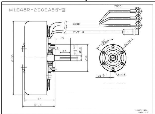
Gambar 8. Dimensi M1048R [4]
