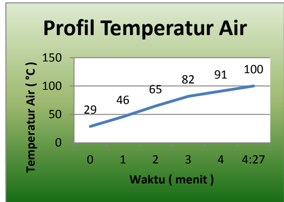
Gambar 5 Grafik Waktu Pendidihan Air
