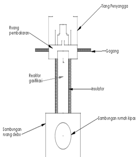
Gambar 2. Model kompor
