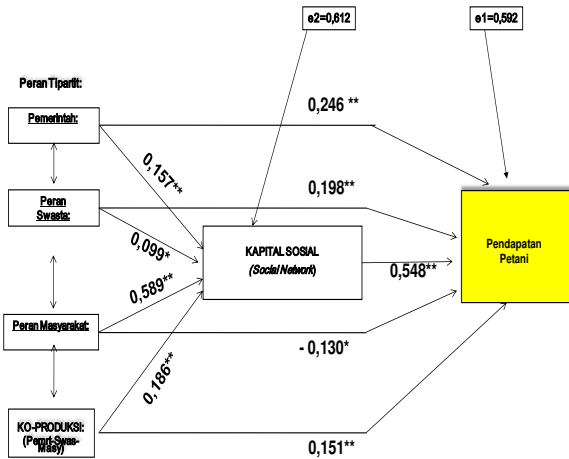
Gambar 2. Hasil akhir analisis jalur hubungan antar variabel
