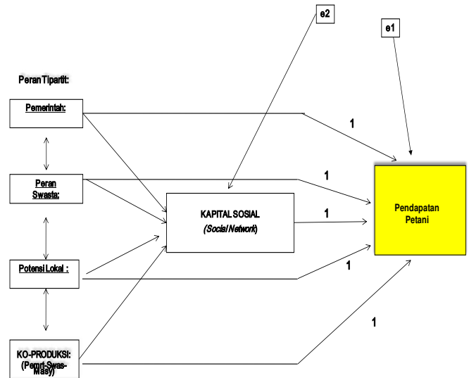
Gambar. 1. Model hipotetik hubungan antara peran tripartit dan koproduksi dengan kapital sosial dan pendapatan
