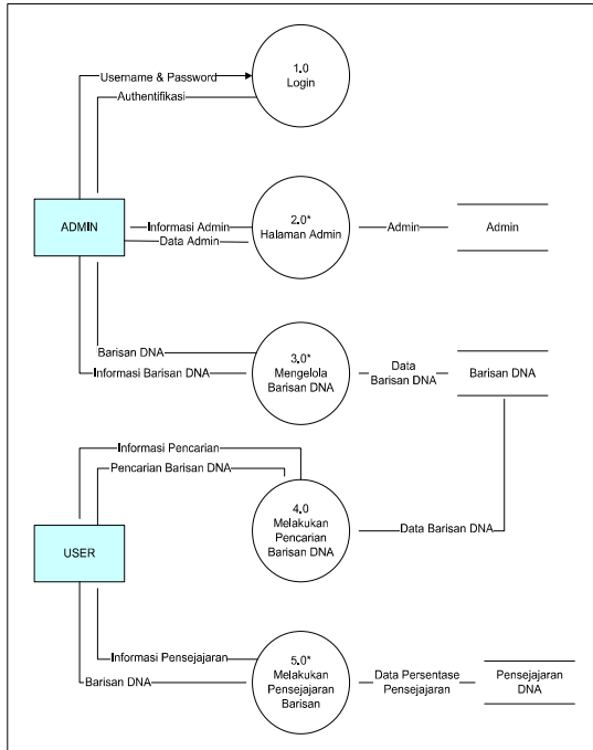
Gambar 3. Diagram Level 1 Sistem penjejajaran Barisan DNA
