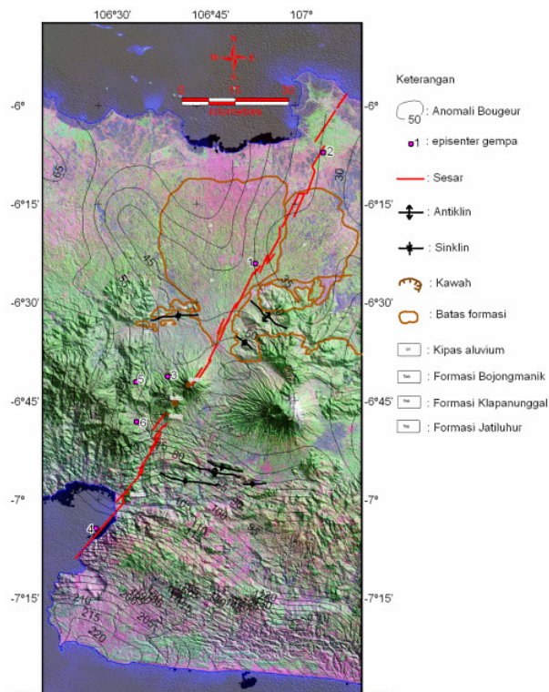
Gambar 5. Sesar Citarik, Tumpang Tindih Citra Landsat, Citra SRTM, Data Anomali Bouguer, Pusat Gempa Bumi dan Hasil Interpretasi Citra[7].
