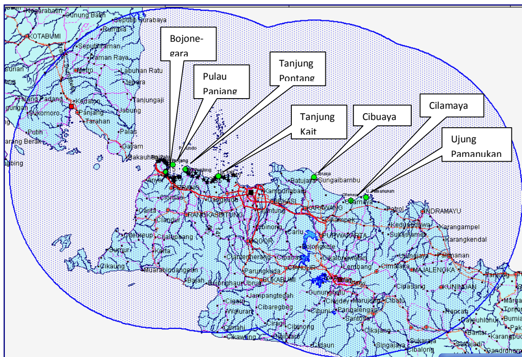
Gambar 1. Peta Wilayah Studi Kegiatan Analisis Regional Jawa Barat dan Banten, Mencakup Daerah-Daerah Interest (●) dan Perluasannya Hingga Radius 150 Km (●).
