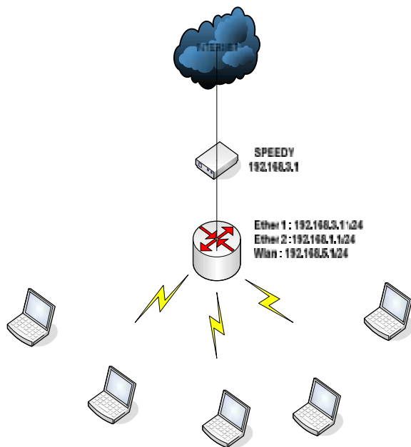
Gambar 4. Rancangan Jaringan Hotspot
