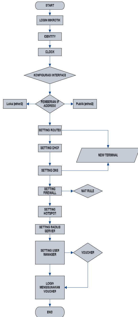
Gambar 5. Flowchart Mikrotik
