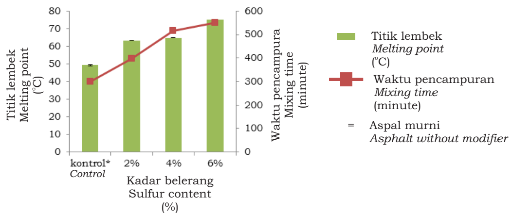
Gambar 1. Pengaruh kadar belerang terhadap titik lembek dan waktu pencampuran aspal modifikasi
