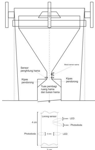
Gambar 4 Penempatan Sensor
