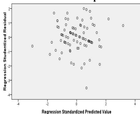
Gambar 3 Grafik Scatterplot
