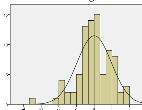
Gambar 1 Grafik Histogram
