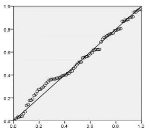
Gambar 2 Grafik Normal
