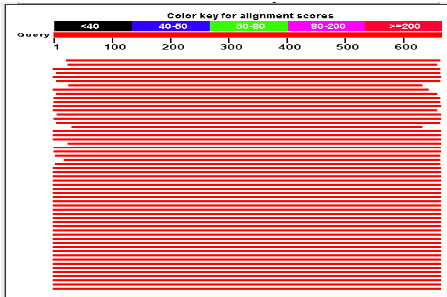
Gambar 4. Tingkat kesamaan sekuen gen CO1 (658 bp) dari serangga laut dengan data di gene bank NCBI ( www.ncbi.nlm.nih.gov ).
