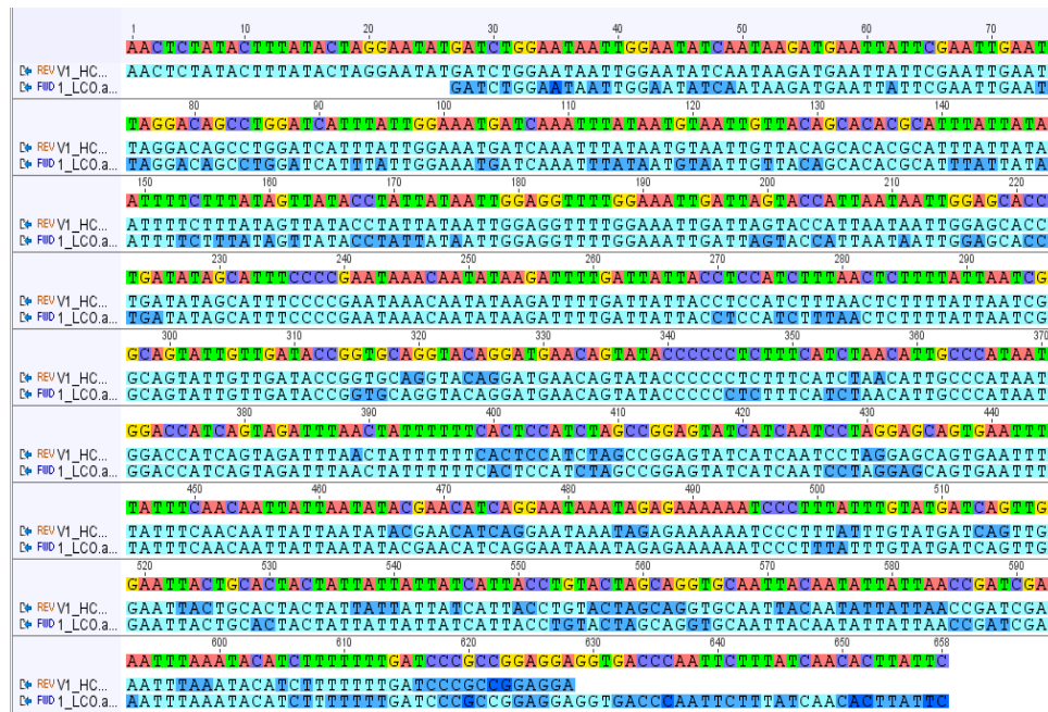
Gambar 3. Konsensus urutan sekuen fragmen DNA serangga laut dengan menggunakan primer CO1
