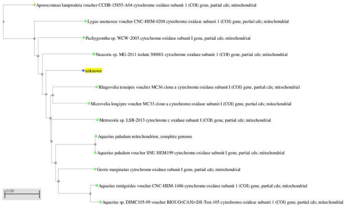
Gambar 5. Pohon filogenetik gen CO1 serangga laut dari perairan Pantai Mokupa dibandingkan dengan data dari NCBI dengan tingkat kemiripan terdekat dan pembanding (outsider).
