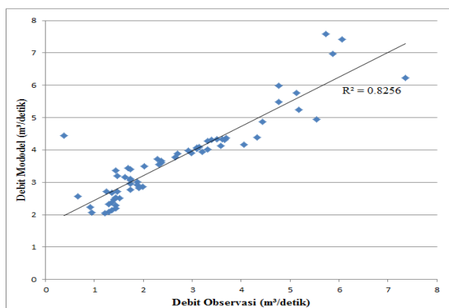
Gambar 4. Hubungan antara debit aliran sungai model dan debit aliran sungai observasi setelah kalibrasi.
