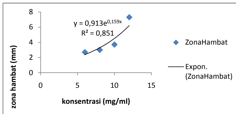
Gambar 2. Korelasi antara Konsentrasi dengan Zona Hambat Ekstrak Gelidium latifolium terhadap C.albicans
