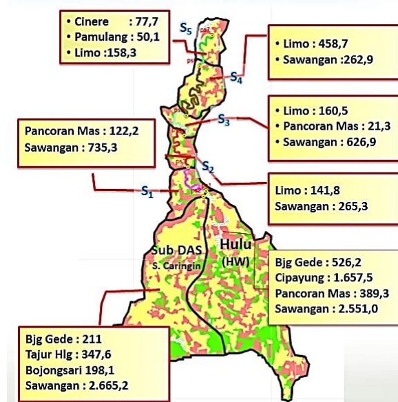
Gambar 5. Peta Potensi Beban Pencemar (PBP) berdasarkan lokasi sumber dan kontribusinya ke setiap segmen di Sungai Pesanggrahan
