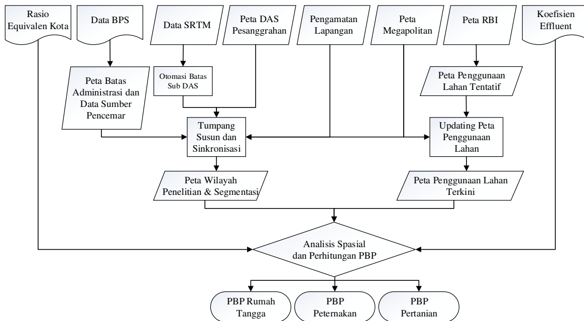
Gambar 1. Diagram alir proses SIG dalam perhitungan potensi beban pencemar
