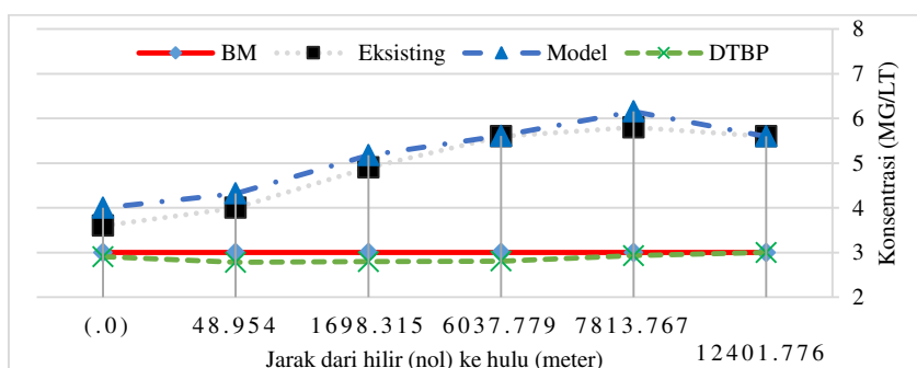
Gambar 6. Grafik kualitas air eksisting, model, DTBP dan baku mutu BOD
