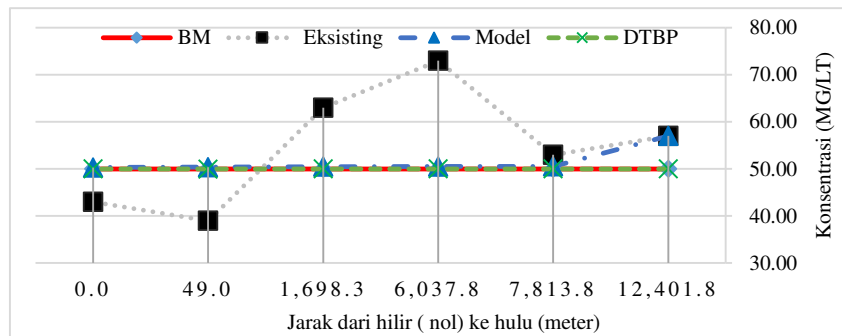
Gambar 8. Grafik kualitas air eksisting, model, DTBP dan baku mutu TSS
