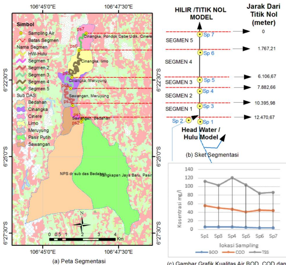
Gambar 4. Peta segmentasi dan zonasi sumber pencemar (Sumber: Analisis SIG dan pengukuran lapangan 2 November 2014)
