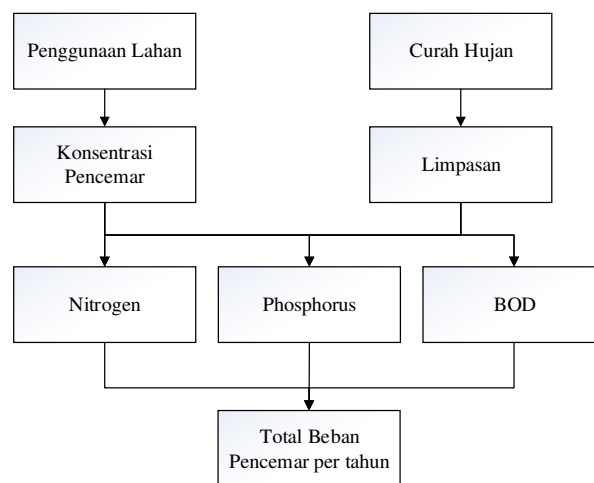
Gambar 2. Model GIS dalam penilaian sumber pencemar Non Point Source (Sumber: Eisakhani (2009))
