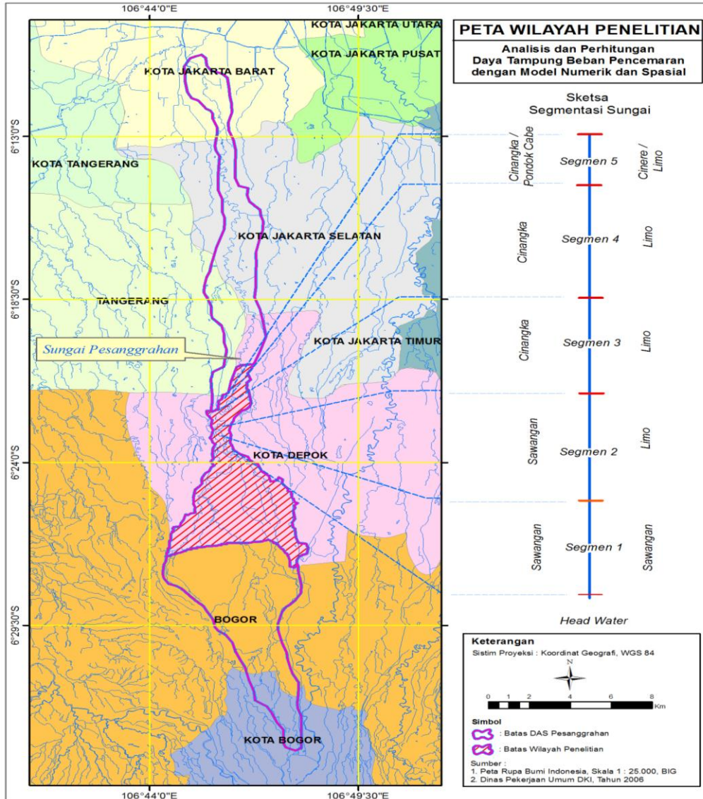
Gambar 1. Peta lokasi Sungai Pesanggrahan dan segmen daerah penelitian di wilayah Depok (Analisis GIS 2014)
