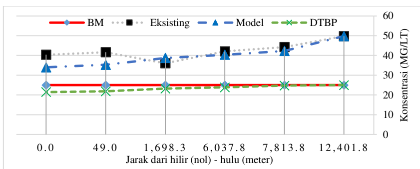
Gambar 7. Grafik kualitas air eksisting, model, DTBP dan baku mutu COD
