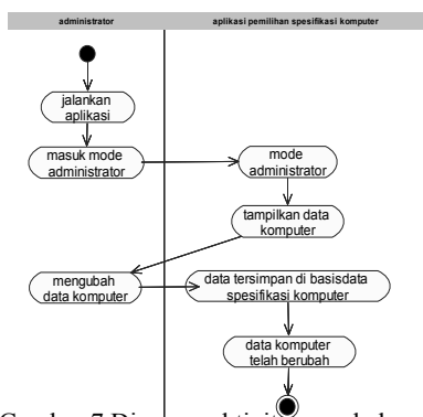
Gambar 7 Diagram aktivitas perubahan data komputer
