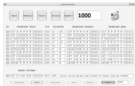
Gambar 9 Hasil iterasi algoritma genetik
