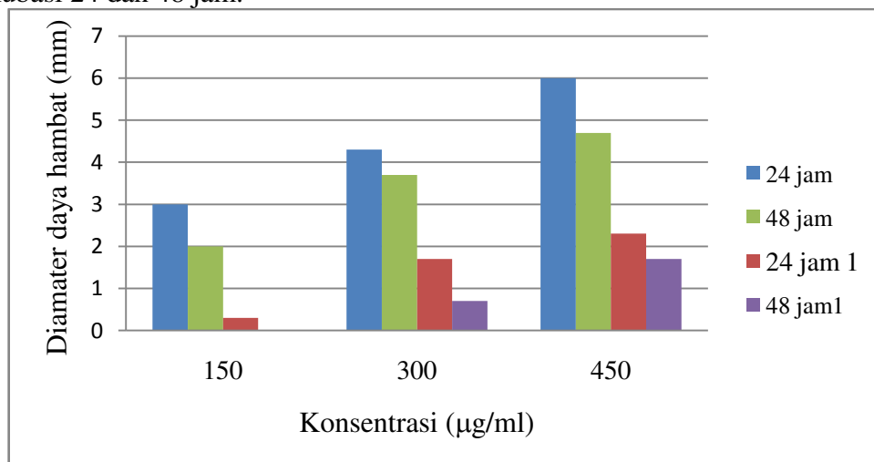
Gambar 2. Diagram Batang Daya Hambat Ekstrak H. scabra setelah Diinkubasi 24 dan 48 Jam terhadap Bakteri P. aeruginosa dan B. Cereus
