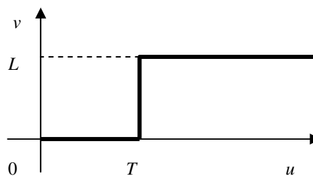
Gambar 2. Operasi pengambangan.
