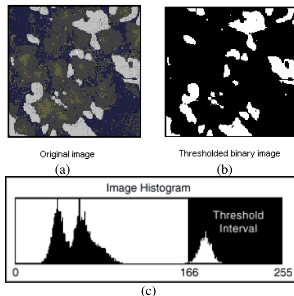
Gambar 3. Segmentasi citra.
