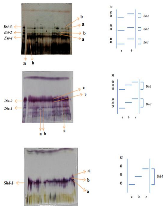
Gambar 2. Zimmogram dan pola berkas pada gel polyacrylamide untuk masing-masing sistem enzim
