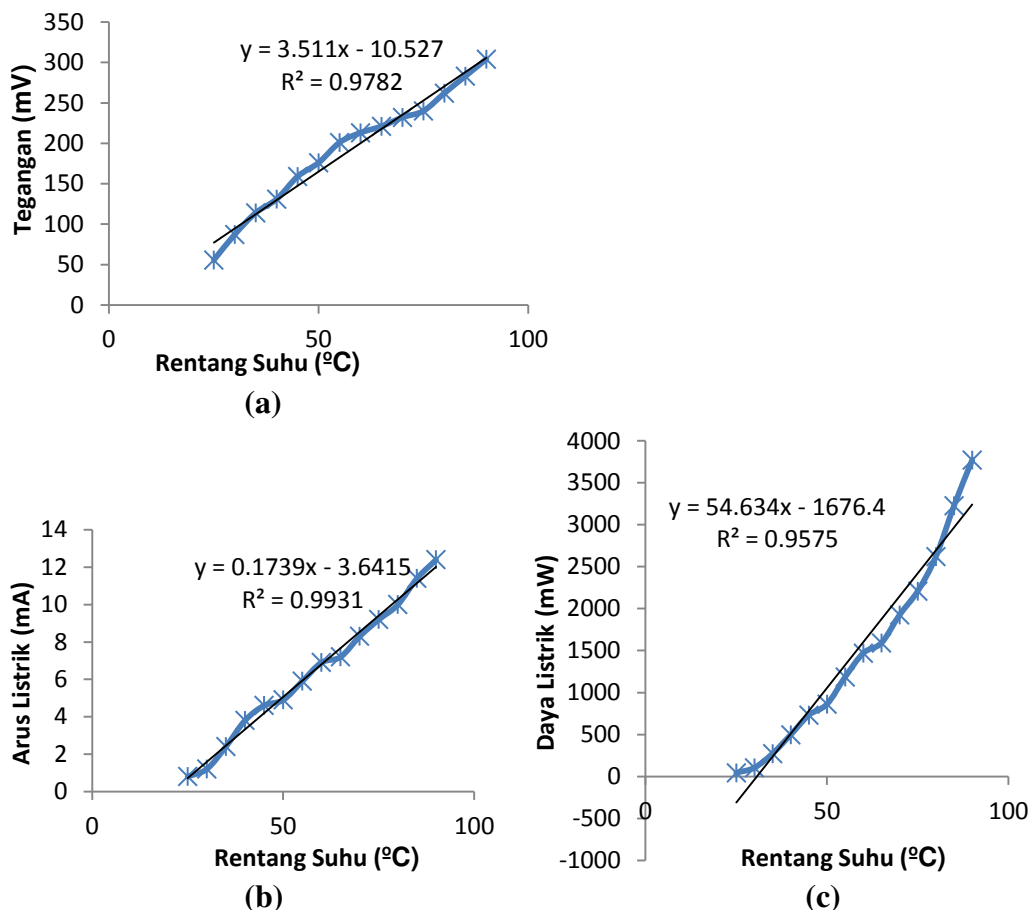
Gambar 1. Grafik Data Hasil Pengukuran; (a) Hubungan Suhu dan Tegangan; (b) Hubungan Suhu dan Arus Listrik; (c) Hubungan Suhu dan Daya Listrik.
