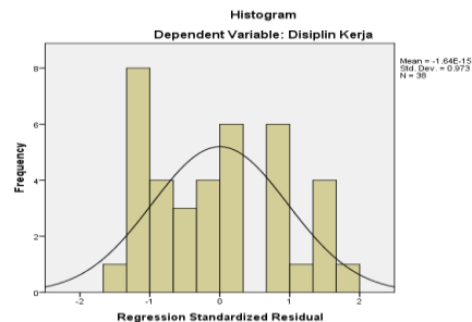
Gambar 2 Kurva Histogram
