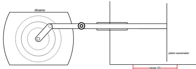
Gambar 2. Konfigurasi Dinamo dan Wavemaker.
