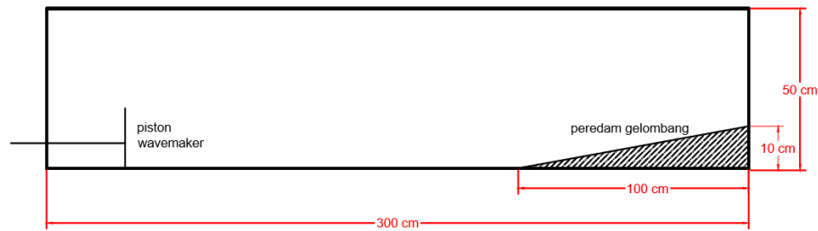
Gambar 1. Penampang Wave Flume Dalam Bidang Dua Dimensi.
