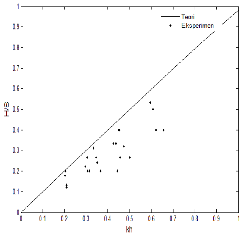
Gambar 4. Grafik kh dan H/S Analitik dan Eksperimen
