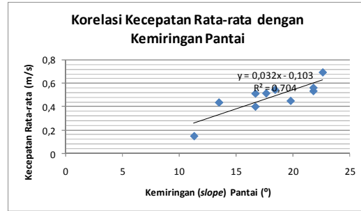
Gambar 9. Korelasi Kecepatan Rata-rata dengan Kemiringan Pantai
