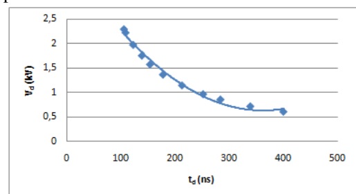
Gambar 12 Karakteristik v-t kaskade arester tanpa elemen dekopling
