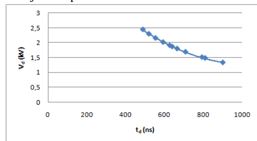
Gambar 8 Karakteristik v-t arrester PCB
