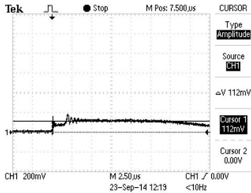
Gambar 15 Pemotongan gelombang tegangan lebih oleh arester PCB pada kaskade arester dengan elemen dekoupling
