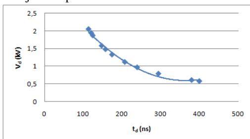
Gambar 10 Karakteristik v-t dioda zener
