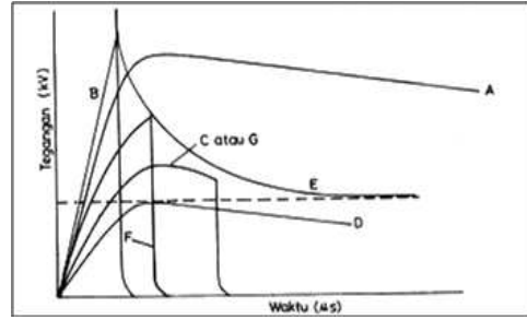
Gambar 3 Karakteristik v-t Sumber: Arismunandar, 1983:115
