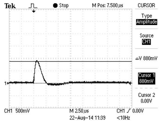
Gambar 14 Pemotongan gelombang tegangan lebih oleh arester PCB pada kaskade arester dengan elemen dekopling
