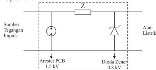
Gambar 7 Objek uji kaskade arrester dengan elemen dekopling
