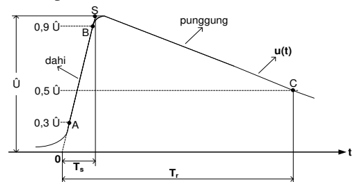
Gambar 5 Parameter tegangan impuls Sumber: Kind, 1993:34
