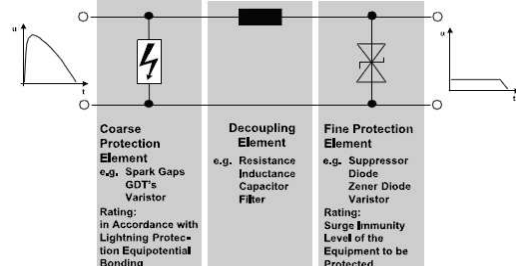
Gambar 4 Rangkaian kaskade arester Sumber: Hasse, 2008:206
