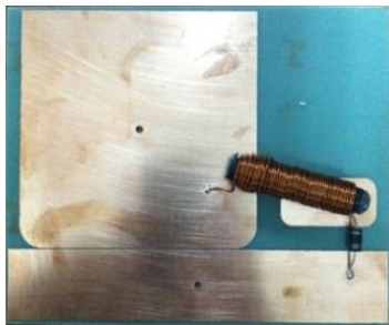
Gambar 11 Kaskade arester dengan elemen dekopling
