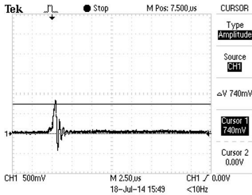
Gambar 9 Pemotongan gelombang tegangan lebih oleh arester PCB
