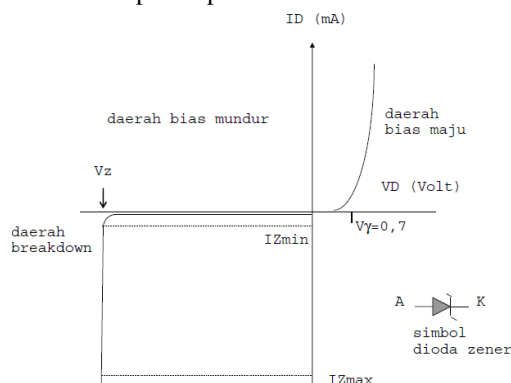
Gambar 1 Kurva karakteristik dioda zener Sumber: Surjono, 2011:42
