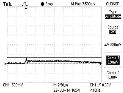
Gambar 11 Pemotongan gelombang tegangan lebih oleh dioda zener
