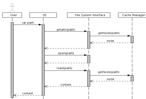
Gambar 9 Sequence Diagram Pembacaan Berkas
