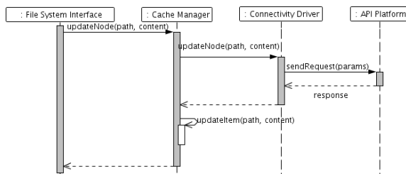
Gambar 4. Sequence Diagram Pemutakhiran Node
