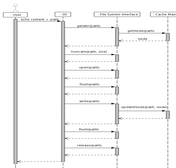
Gambar 10 Sequence Diagram Penulisan Berkas
