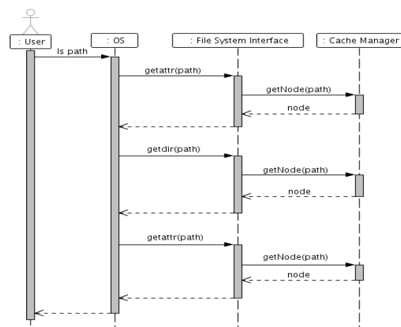
Gambar 8. Sequence Diagram Penampilan Isi Direktori
