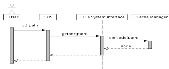
Gambar 7 Sequence Diagram Perpindahan Direktori melalui driver yang digunakan (lihat Gambar 3).
