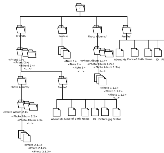
Gambar 2. Hirarki Sistem Berkas Sniffs
