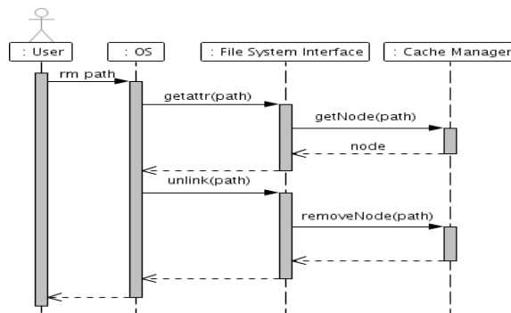
Gambar 11 Sequence Diagram Penghapusan Berkas
