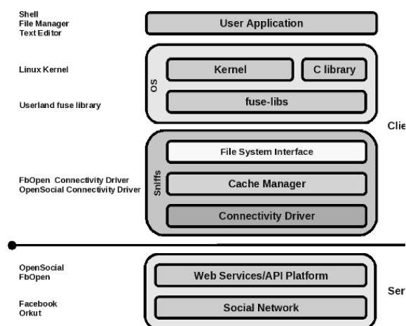
Gambar 1. Arsitektur Sniffs
