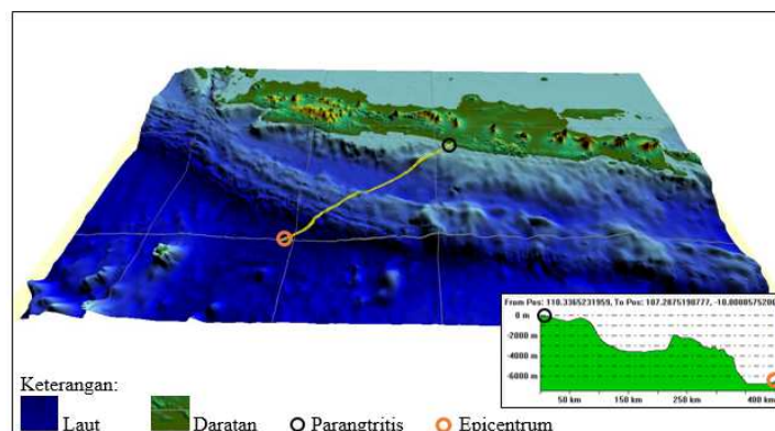
Gambar 4. Morfologi Dasar Laut Daerah Istimewa Yogyakarta
