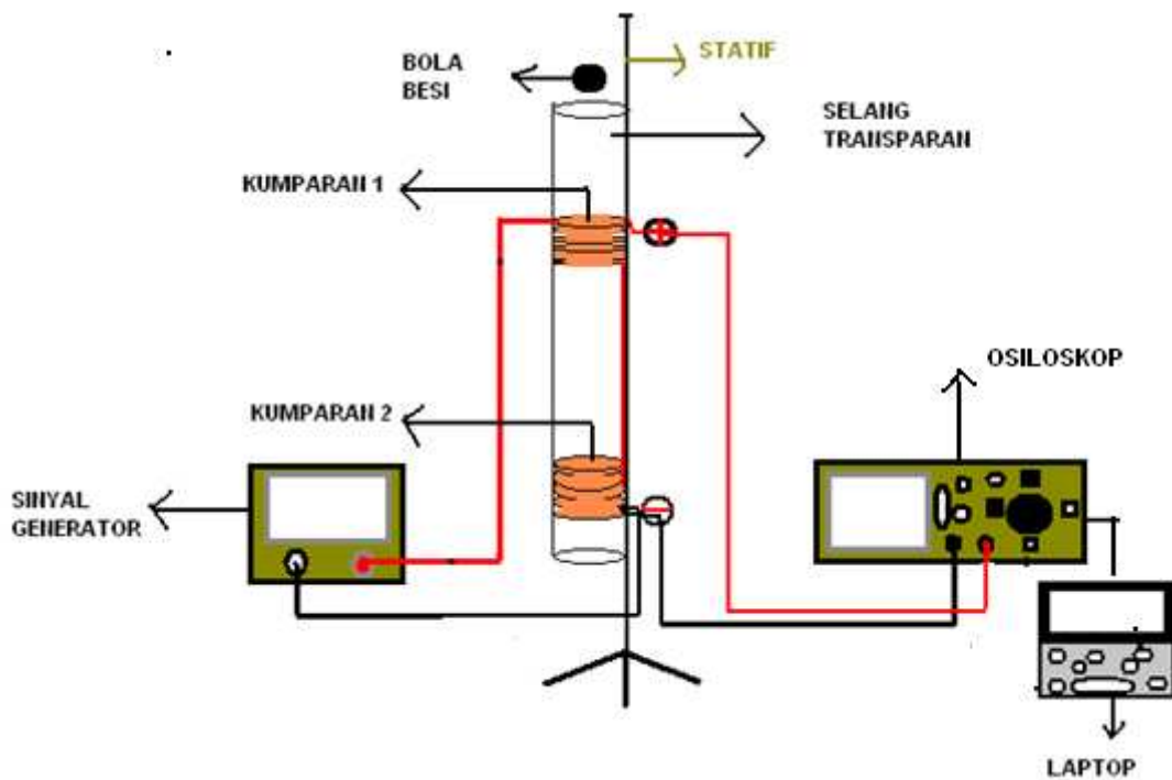
Gambar 3. Rancangan alat
