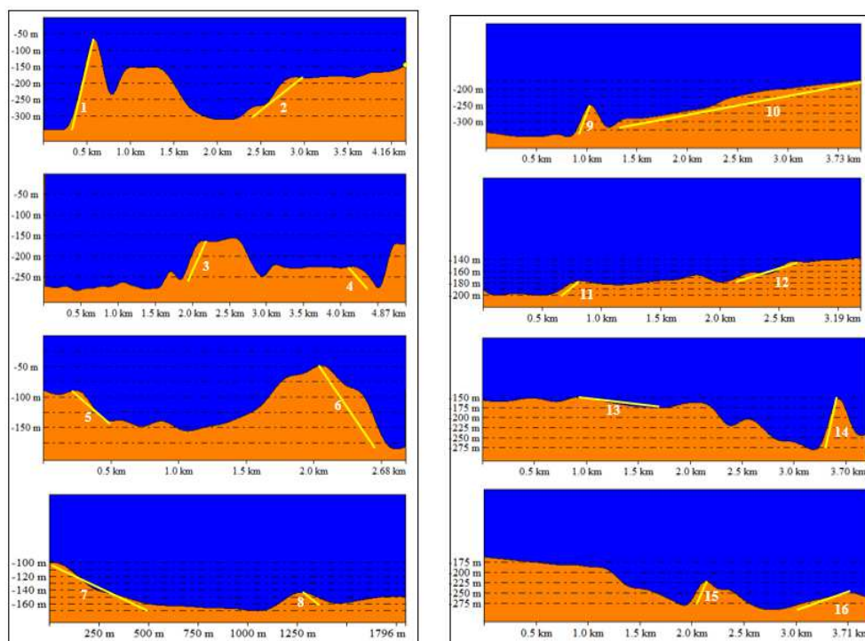
Gambar 7. Bentuk Morfologi Dasar Laut Perairan Pulau Komodo (Pengolah Data Penelitian, 2013).
