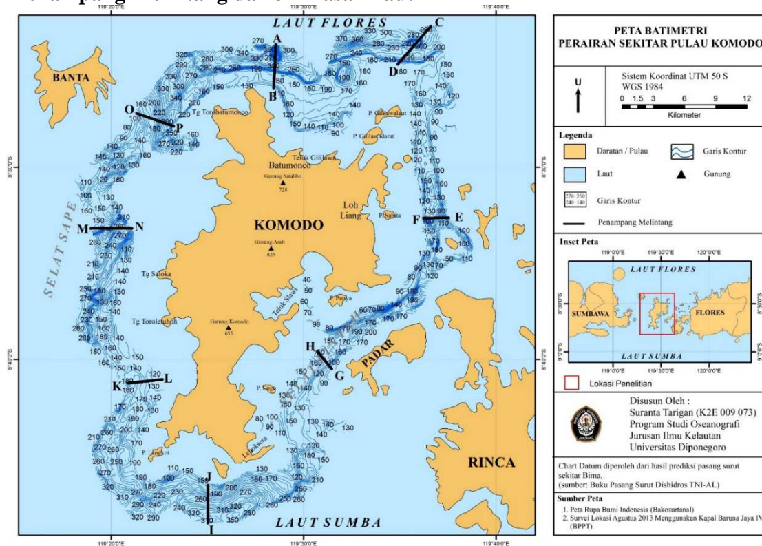
Gambar 6. Peta Batimetri dengan Garis Penampang Melintang (Pengolahan Data Lapangan, 2013).
