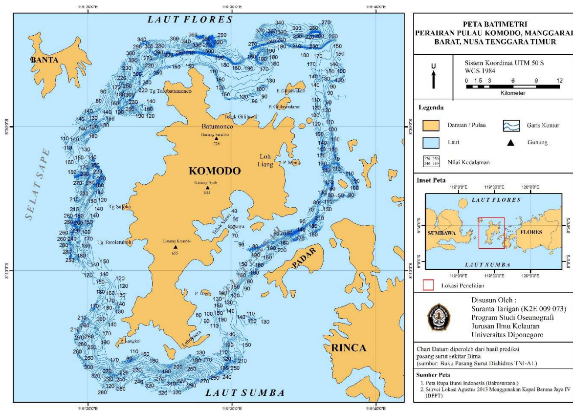
Gambar5.PetaBatimetriPerairanPulau Komodo (Pengolahan Data Lapangan, 2013).
