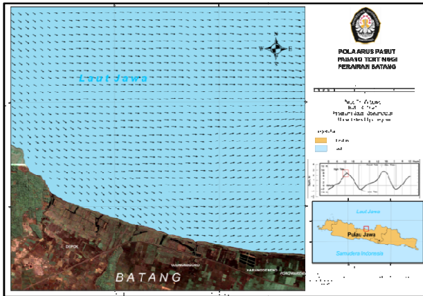
Gambar 5. Pola arus pasut saat pasang tertinggi perairan Batang
