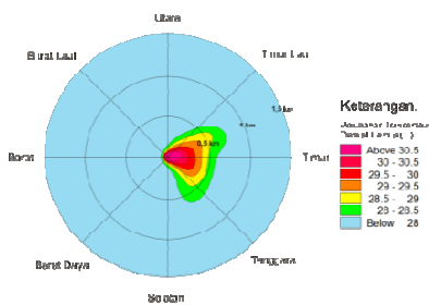
Gambar 21. Radius sebaran panas saat pasang tertinggi pada pasang perbani
