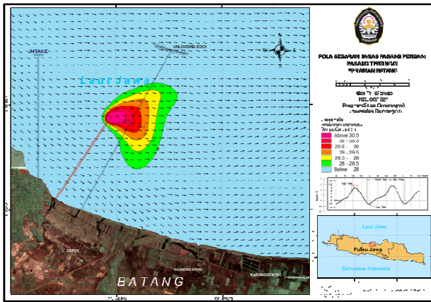
Gambar 17. Pola sebaran panas pasang perbani saat pasang tertinggi pada perairan Batang
