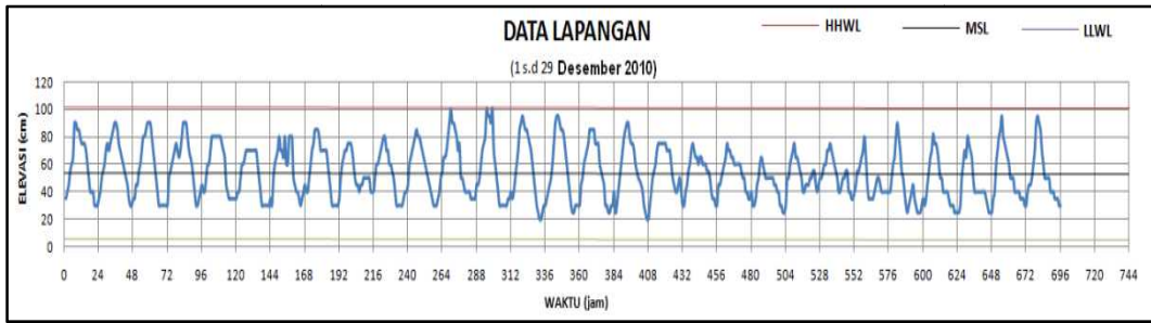
Gambar 4. Grafik pasang surut hasil pengukuran lapangan
