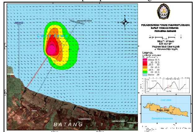
Gambar 12. Pola sebaran panas pasang purnama saat surut menuju pasang pada perairan Batang
