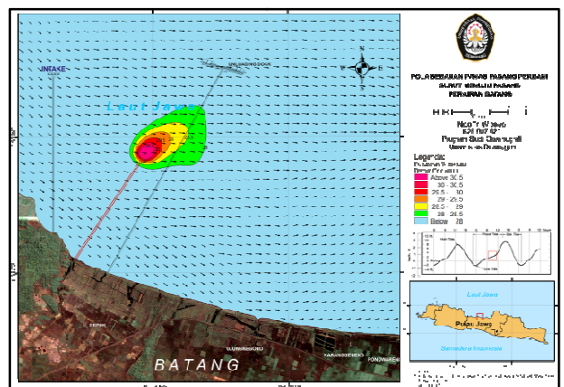
Gambar 20. Pola sebaran panas pasang perbani saat surut menuju pasang pada perairan Batang
