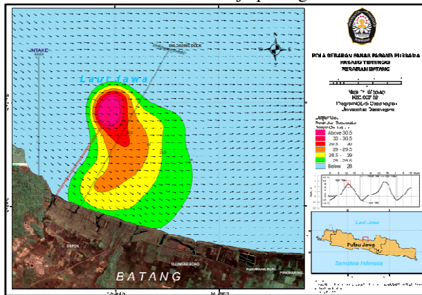
Gambar 9. Pola sebaran panas pasang purnama saat pasang tertinggi pada perairan Batang
