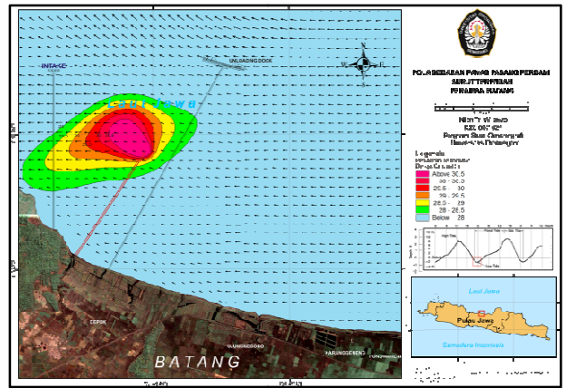
Gambar 19. Pola sebaran panas pasang perbani saat surut terendah pada perairan Batang
