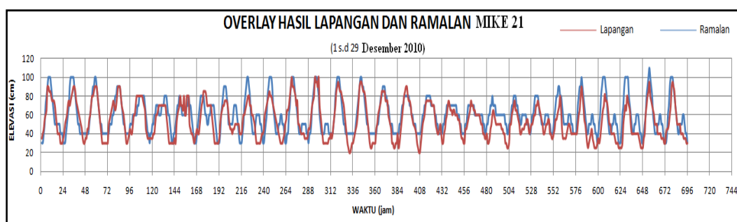
Gambar 25. Grafik overlay pasang surut lapangan dan ramalan MIKE 21
