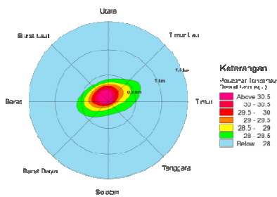
Gambar 22. Radius sebaran panas saat pasang menuju surut pada pasang perbani
