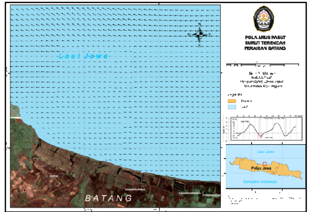
Gambar 7. Pola arus pasut saat surut terendah perairan Batang
