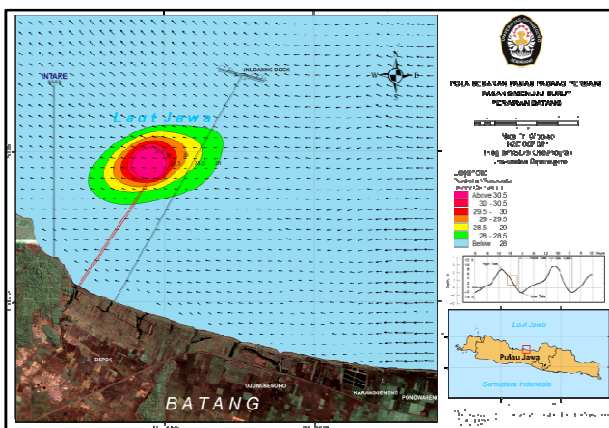
Gambar 18. Pola sebaran panas pasang perbani saat pasang menuju surut pada perairan Batang
