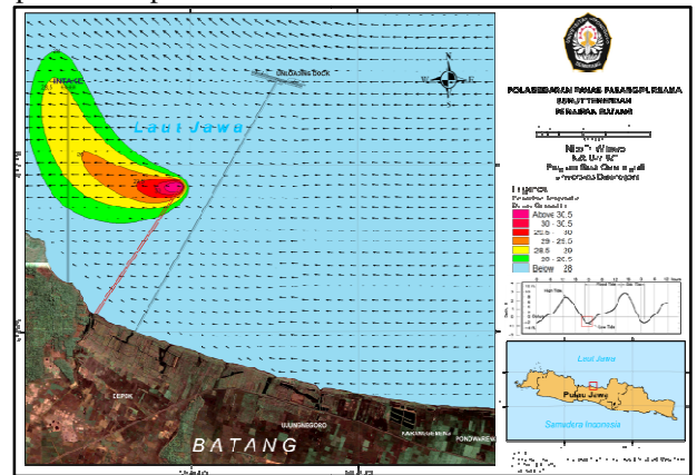
Gambar 11. Pola sebaran panas pasang purnama saat surut terendah pada perairan Batang
