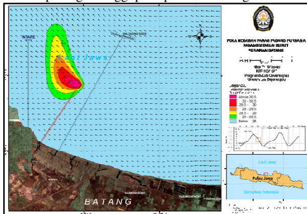
Gambar 10. Pola sebaran panas pasang purnama saat pasang menuju surut pada perairan Batang
