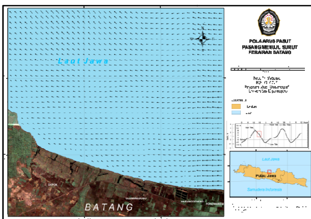
Gambar 6. Pola arus pasut saat pasang menuju surut perairan Batang
