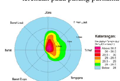
Gambar 16. Radius sebaran panas saat surut menuju pasang pada pasang purnama
