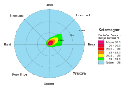
Gambar 24. Radius sebaran panas saat surut menuju pasang pada pasang perbani
