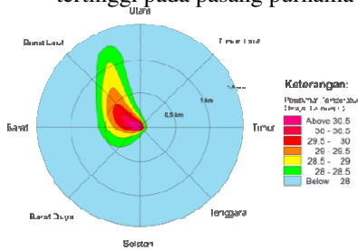
Gambar 14. Radius sebaran panas saat pasang menuju surut pada pasang purnama
