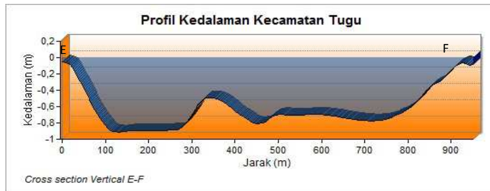
Gambar 6. Profil Kedalaman Tegak Lurus Pantai (E-F)
