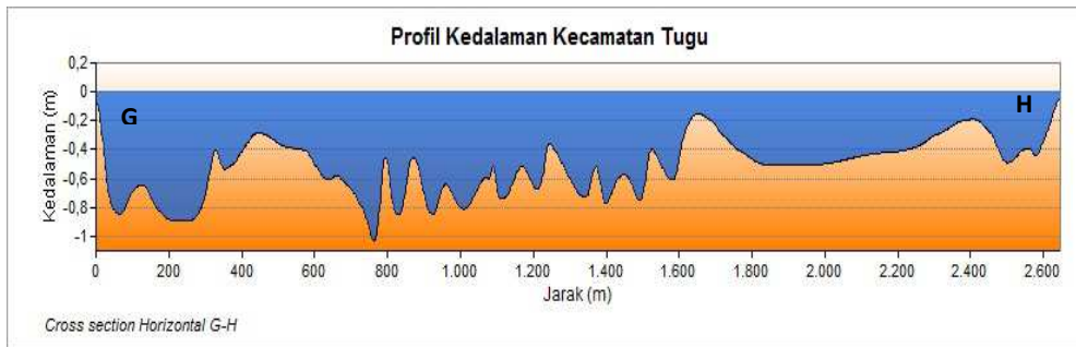
Gambar 7. Profil Kedalaman Sejajar Pantai (G-H)
