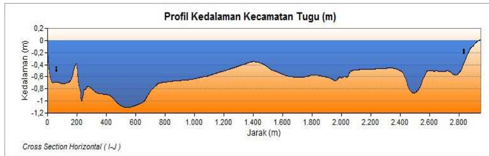
Gambar 8. Profil Kedalaman Sejajar Pantai (i-j)
