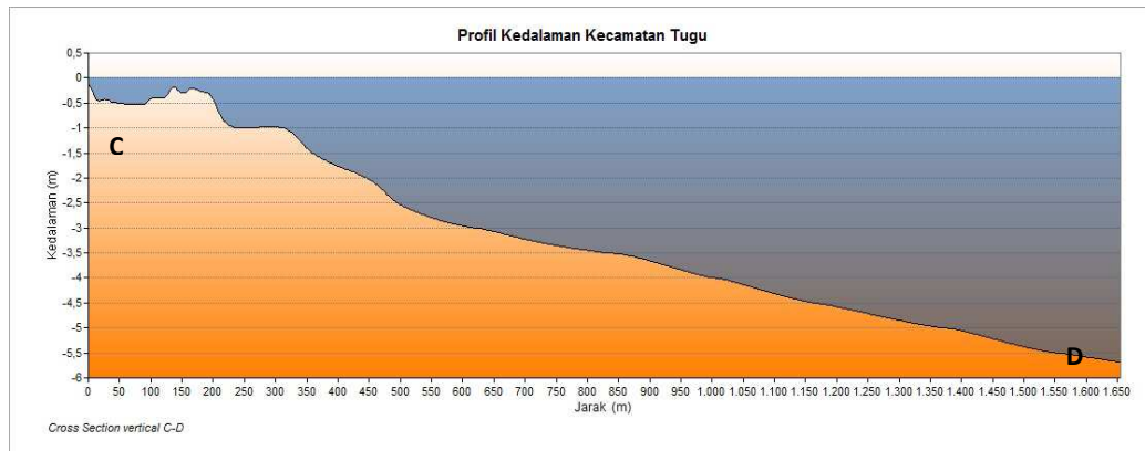
Gambar 5. Profil Kedalaman Tegak Lurus Pantai (C-D)
