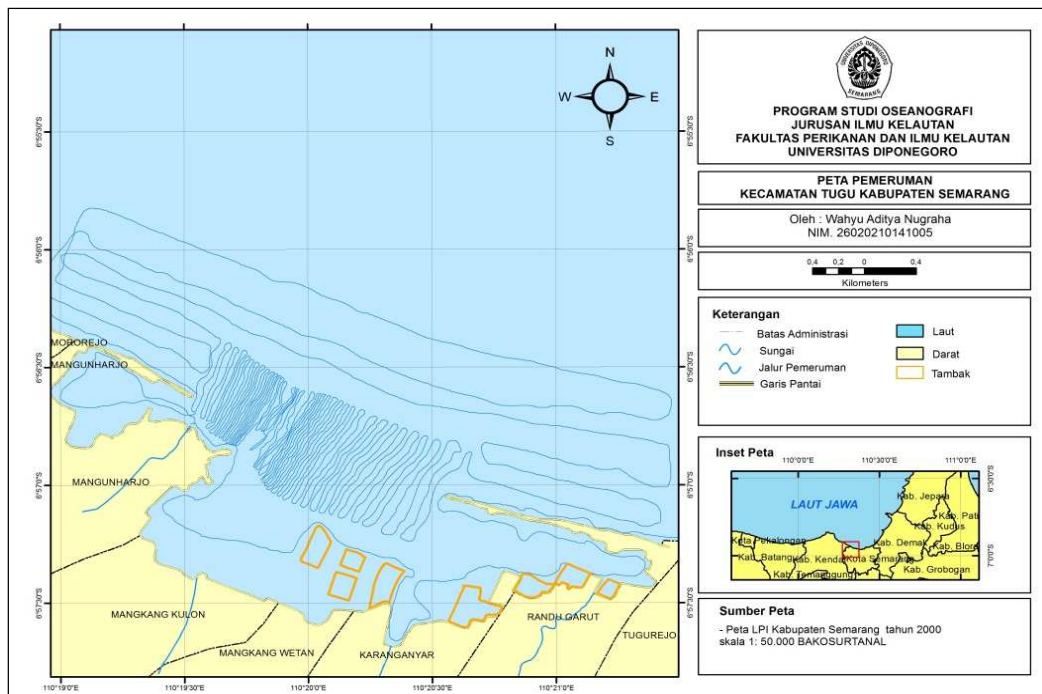
Gambar 1. Hasil Jalur Pemeruman
