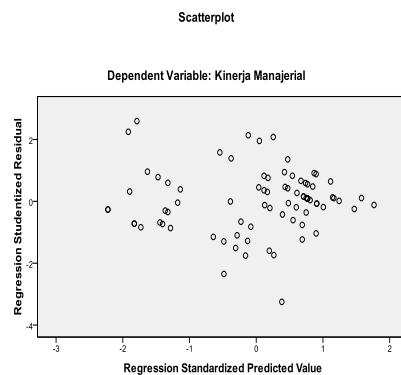
Gambar 2 Uji Heteroskedastisitas
