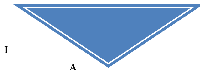
Gambar 1. Sistem vokal minimal; Jakobson dalam Soenjono (2000)
