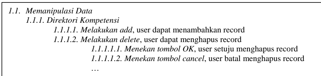
Gambar 5. Spesifikasi Pekerjaan Pengguna
