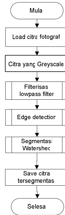
Gambar 4. Detail Desain Aplikasi
