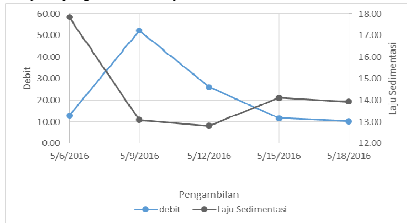
Gambar 4. Grafik hubungan debit sungai dengan laju sedimentasi
