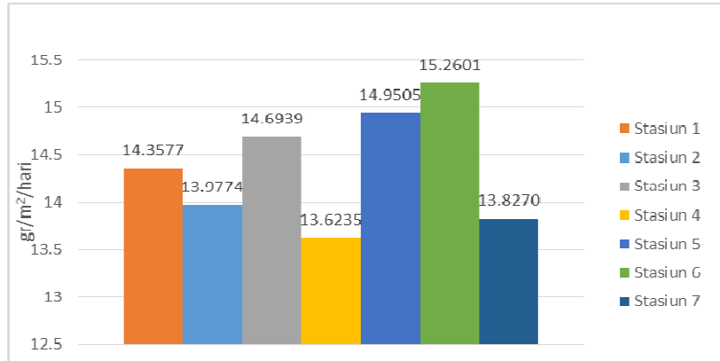
Gambar 3. Rata – rata laju sedimentasi tiap stasiun
