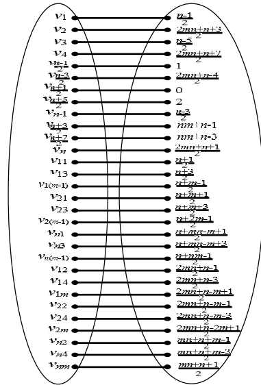
Gambar 12 Pemetaan bijektif g pada graf korona
