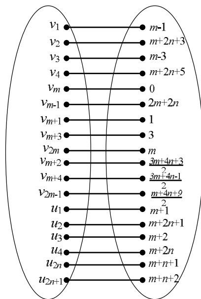
Gambar 5 Pemetaan bijektif g pada graf C_{2m} @ K_{1, 2n+1} dengan m bilangan ganjil
