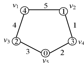
Gambar 2 Pelabelan graceful sisi pada graf C5
