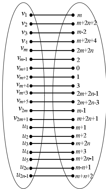
Gambar 9 Pemetaan bijektif g pada graf C_{2m+1} @ K_{1,2n} untuk m bilangan genap
