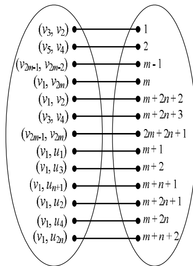
Gambar 4 Pemetaan bijektif f pada graf C_{2m} @ K_{1, 2n+1}
