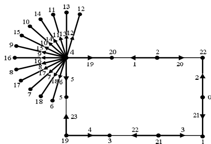
Gambar 7 C_{10} @ K_{1,13} dengan pelabelan graceful sisi berarah
