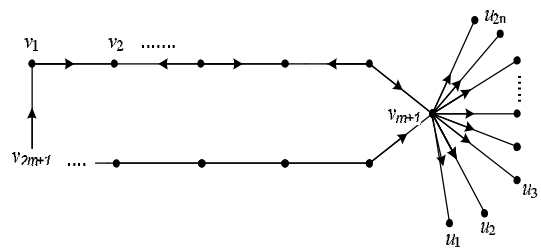
Gambar 8 Graf C_{2m+1} @ K_{1,2n} yang semua sisinya telah diberi arah
