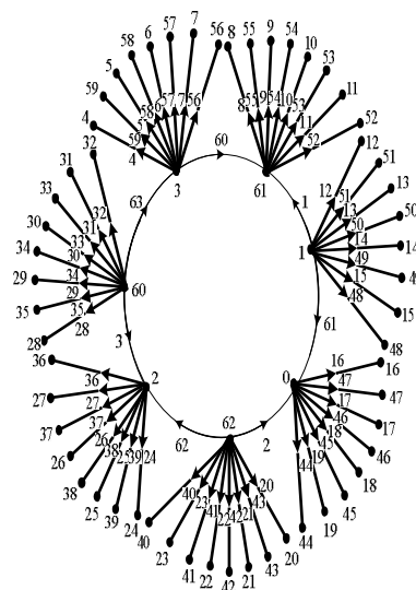
Gambar 13 Graf C_7 \odot \bar{K}_8 dengan pelabelan graceful sisi berarah
