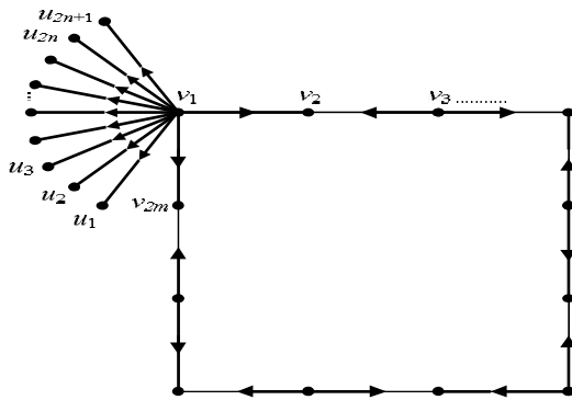
Gambar 3 Graf C_{2m} @ K_{1, 2n+1} yang semua sisinya telah diberi arah
