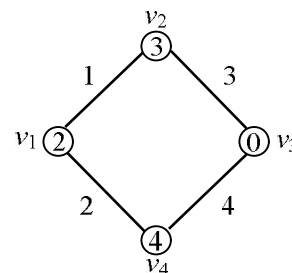
Gambar 1 Pelabelan graceful pada graf C4
