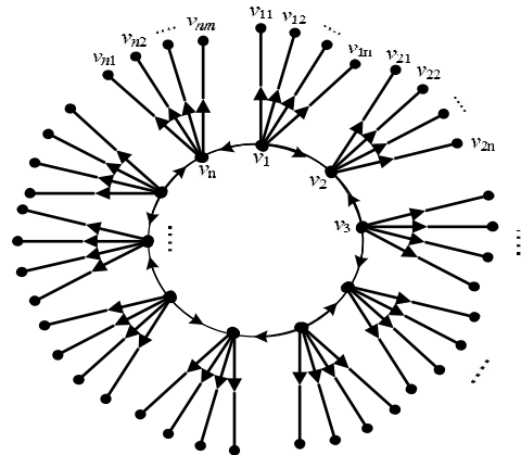
Gambar 11 Graf Korona C_n @ \bar{K}_m yang sisi-sisinya telah diberi arah
