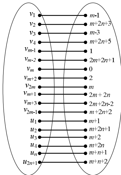
Gambar 6 Pemetaan bijektif g pada graf C_{2m} @ K_1 , 2n+1 dengan m bilangan genap
