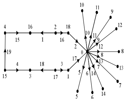
Gambar 10 Graf C_9 @ K_{1,10} dengan pelabelan graceful sisi berarah
