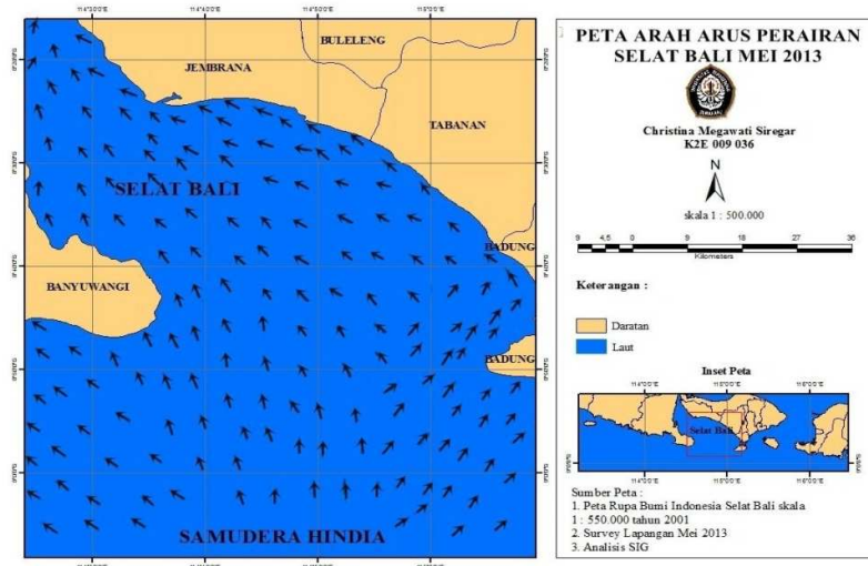
Gambar 6. Peta Arah Arus Di Perairan Selat Bali bagian Selatan
