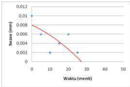
Gambar 4.12 Hubungan Tinggi sampel terhadap Waktu untuk Menentukan Ps i, Tanah Dengan Kadar Kapur 8%
