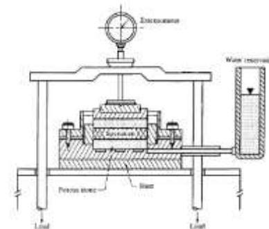
Gambar 2.21 Alat uji Konsolidasi (konsolidometer)
