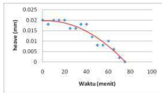
Gambar 4.10 Hubungan Tinggi sampel terhadap Waktu untuk Menentukan P_s i, Tanah Dengan Kadar Kapur 6%
