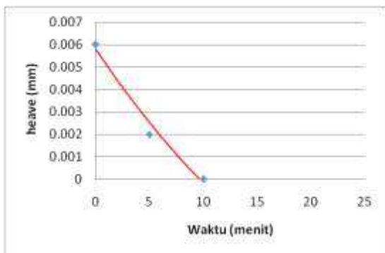
Gambar 4.12 Hubungan Tinggi sampel terhadap Waktu untuk Menentukan Ps i, Tanah Dengan Kadar Kapur 10%
