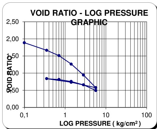
Gambar 4.5 Void Rasio dengan Log Pressure
