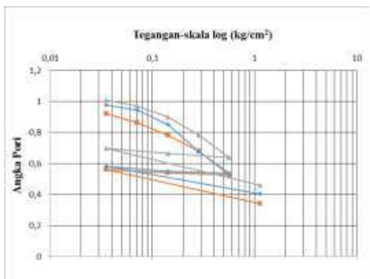
Gambar 4.9 Void Rasio dengan Log Pressure campuran Kapur 6%, 8%, 10%
