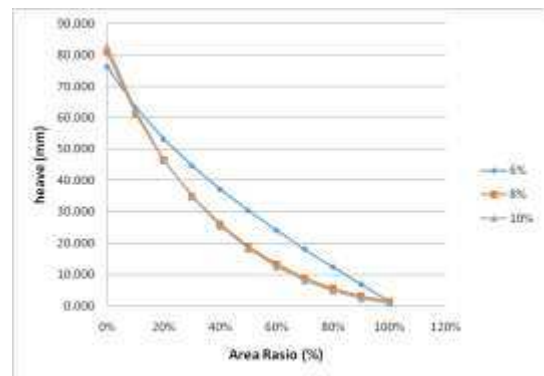
Gambar 4.17 Hubungan Rasio Luas dengan Heave, Tanah Prosentase Kapur 6%, 8%, 10%
