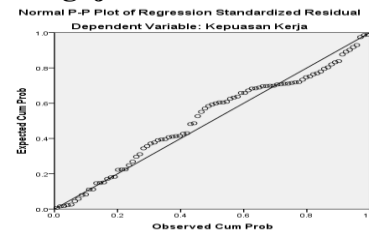
Gambar 1 Hasil Pengujian Normalitas Data
