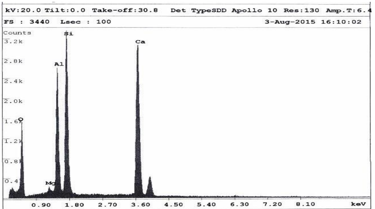
Gambar 2 Hasil karakterisasi menggunakan SEM-EDX untuk sampel 2
