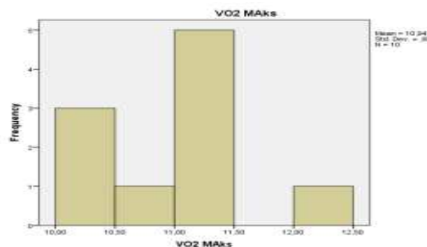
Gambar 2. Histogram tingkat volume oksigen maksimal ( VO_2 Max)
