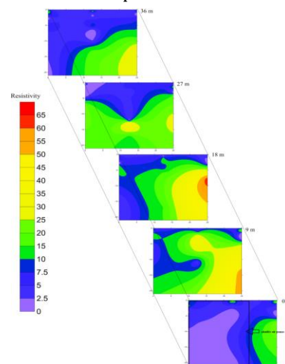
Gambar 4. Penampang vertikal kedalaman lapisan bawah permukaan
