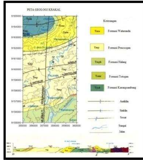
Gambar 2. Peta geologi daerah Krakal
