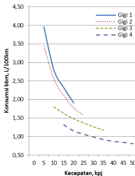
Gambar 3 Konsumsi bbm Pertamax Plus pada berbagai posisi gigi
