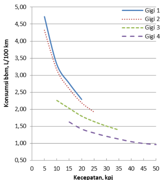
Gambar 1 Konsumsi bbm Premium pada berbagai posisi gigi
