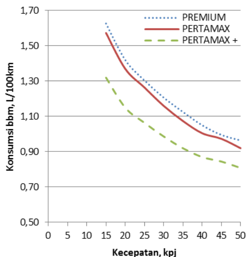
Gambar 7 Konsumsi bahan bakar pada posisi gigi 3
