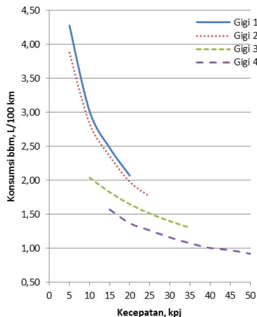
Gambar 2 Konsumsi bbm Pertamax pada berbagai posisi gigi
