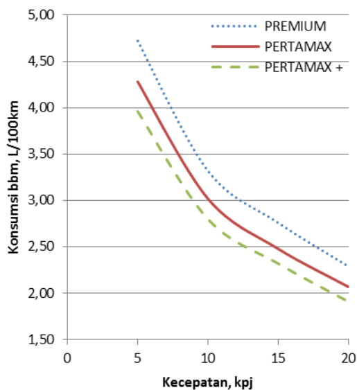
Gambar 4 Konsumsi bahan bakar pada posisi gigi 1
