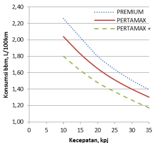
Gambar 6 Konsumsi bahan bakar pada posisi gigi 3
