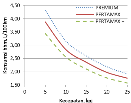
Gambar 5 Konsumsi bahan bakar pada posisi gigi 2
