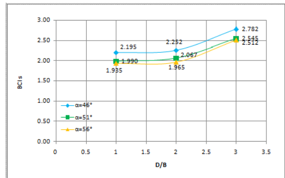
Gambar 5. Grafik Perbandingan Peningkatan (BCIs) Pada s/B = 2% Dengan Variasi Jarak Pondasi dan Sudut Kemiringan Lereng
