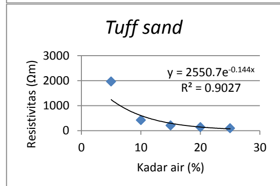
Gambar 9. Hubungan nilai resistivitas dengan kadar air untuk tiap jenis tanah
