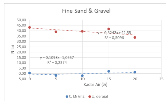
Gambar 4 Grafik hubungan kadar air terhadap phi ( \phi ) dan kohesi pada Fine Sand & Gravel
